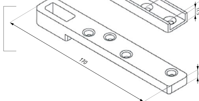
Ramię dolne Door strap
