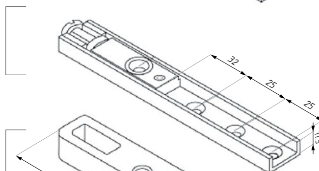
Płytki z regulowaną osią Adjustable top centre
