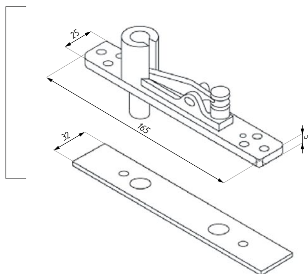
Płytki z regulowanym trzcieniem Walking pivot c/w s.s plate
